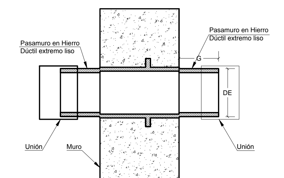
DETALLE N° 4 - PASAMUROS TIPO C TRAMOS HORIZONTALES CON PROLONGACIÓN A AMBOS LADOS DEL MURO ESCALA 1:10
