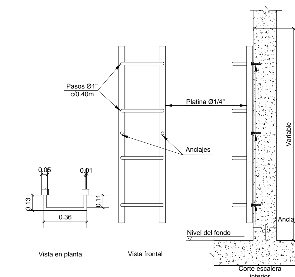
DETALLE N°1 ESCALERA UÑA DE GATO ESCALA 1:20
