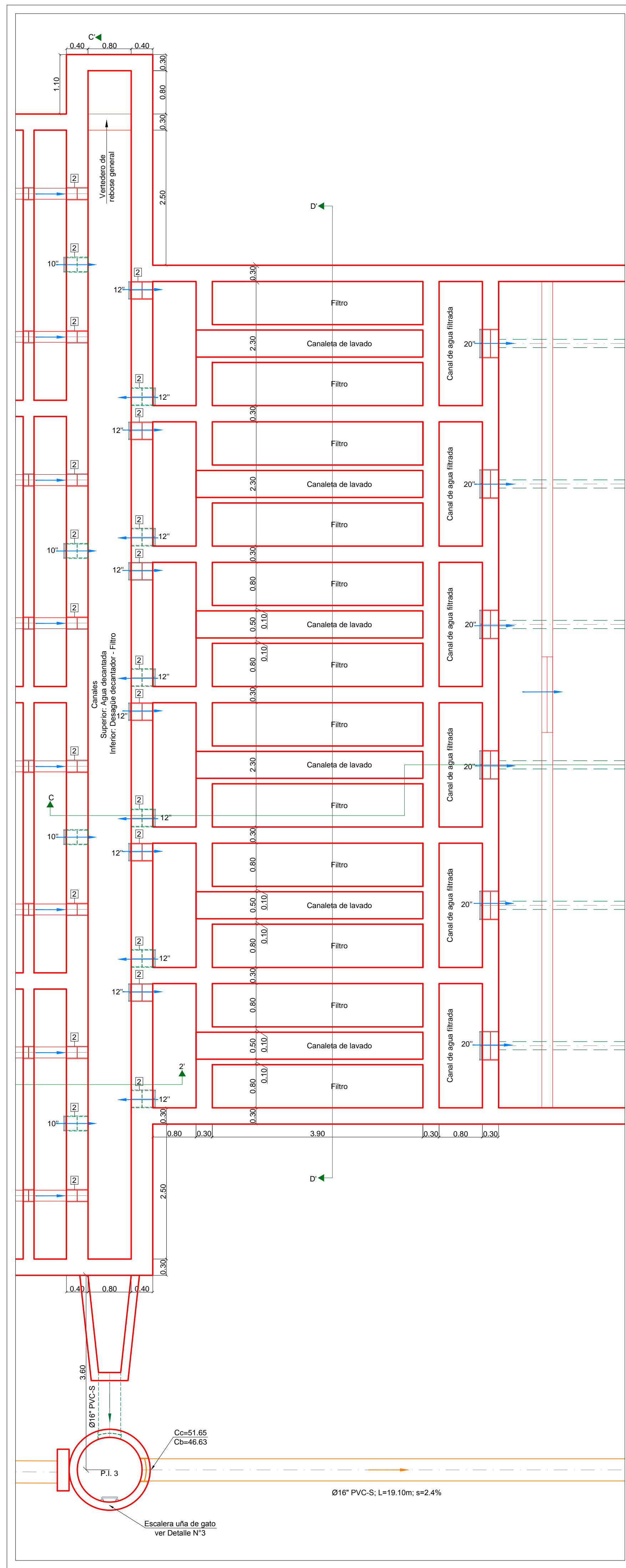
PLANTA FILTRO ESCALA 1:50
