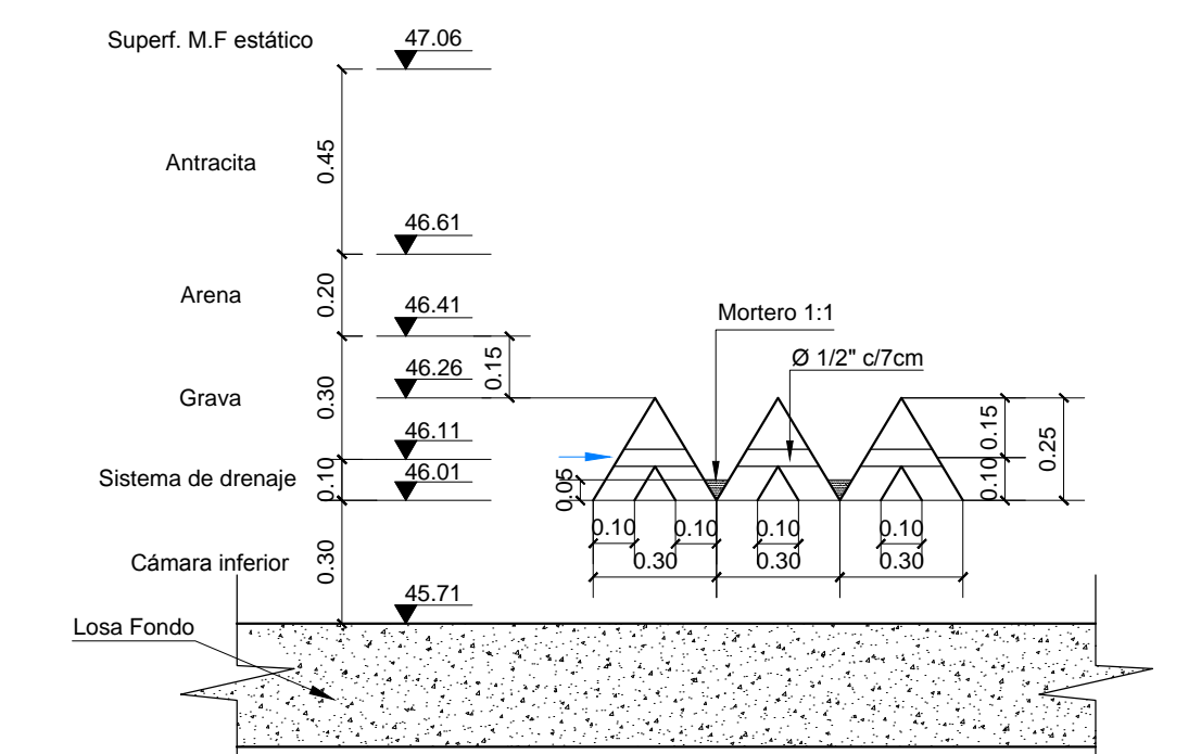
DETALLE N°2 SISTEMA DE DRENAJE DE FILTROS ESCALA 1:20
