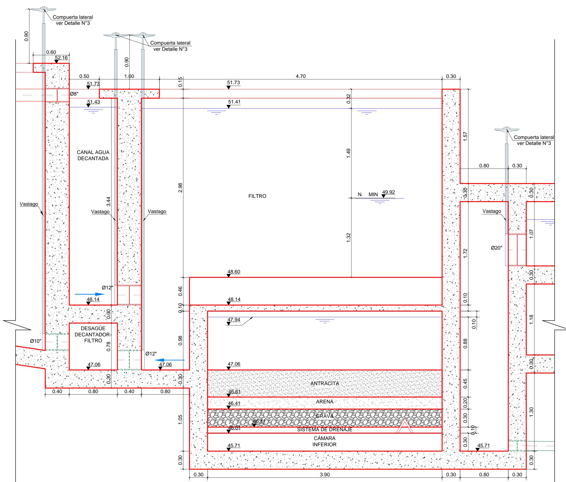
CORTE C-C' FILTRO ESCALA 1:30
