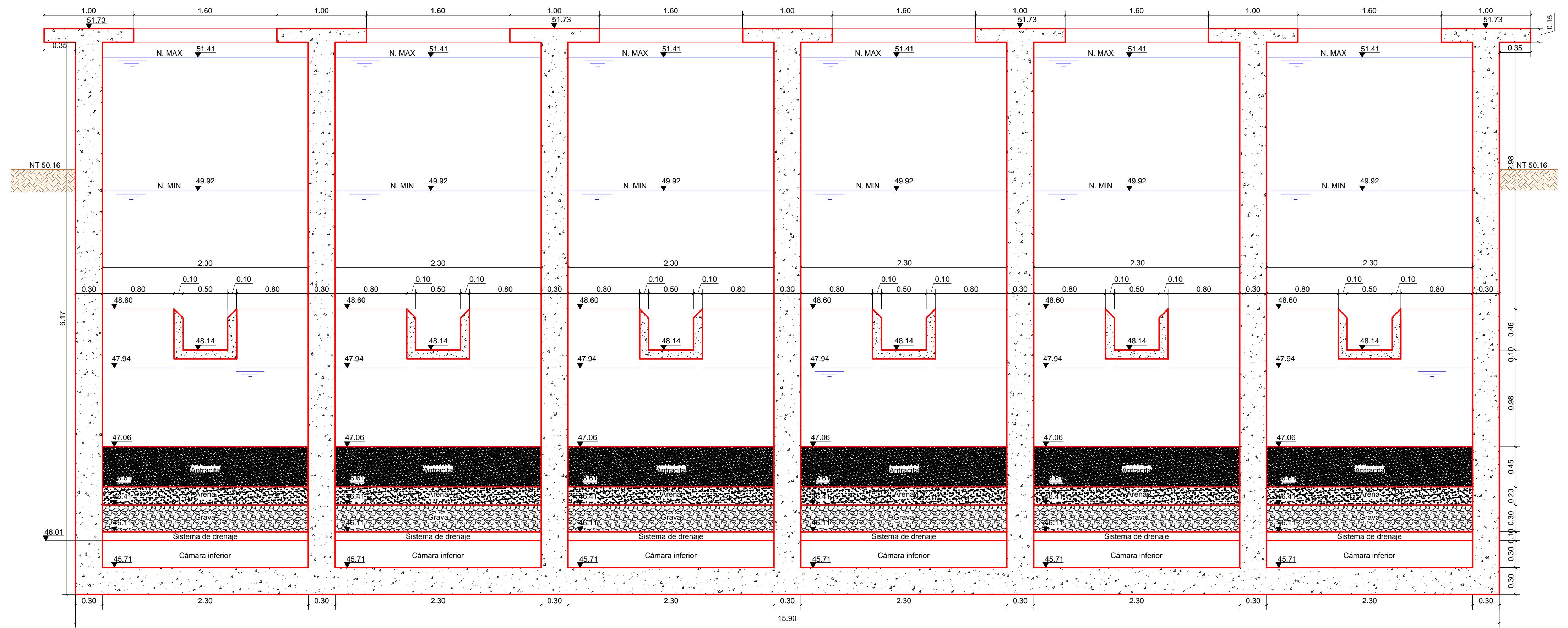
CORTE D-D' FILTRO ESCALA 1:30
