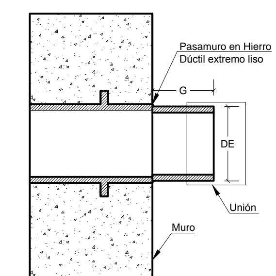
DETALLE N° 4 - PASAMUROS TIPO B HACIA UN COSTADO DEL MURO ESCALA 1:10
